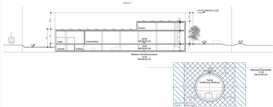
Abb. 2 Lage der Tunnelröhre in Bezug auf den Neubau (Querschnitt senkrecht zu den Bahngeleisen)
