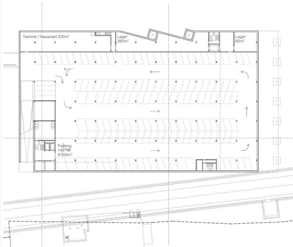
Abb. 3 Verlauf der Tunnelröhre (unterer Bildrand)
