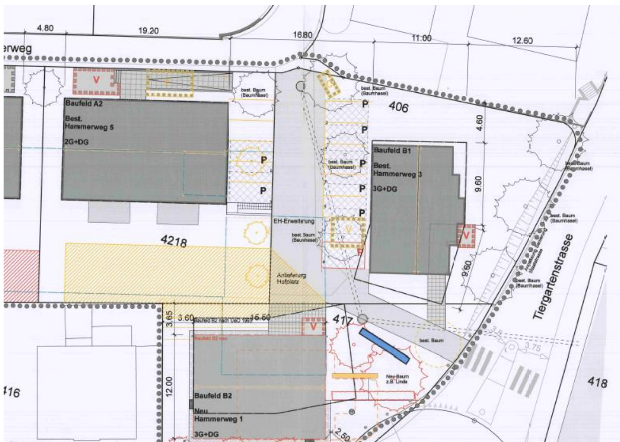
Auszug UeO Hammerweg
