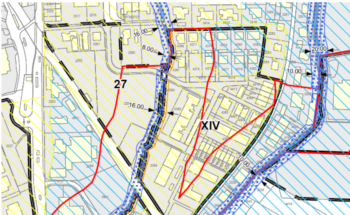
Auszug Zonenplan 3 – UeO Bürgergasse I
