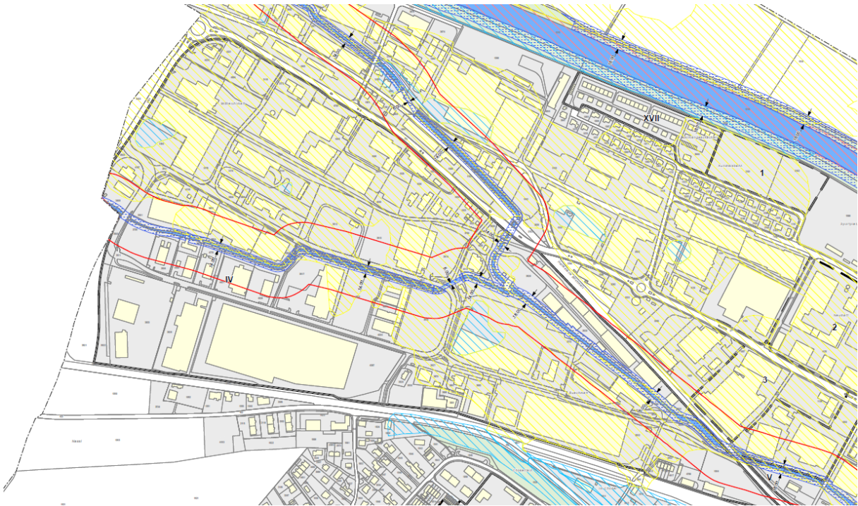
Auszug Zonenplan 3 – UeO Industrie Buchmatt
