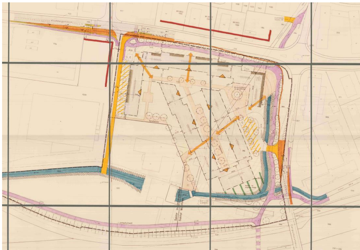
Auszug UeO Tiergarten
